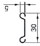
夹板截面图
